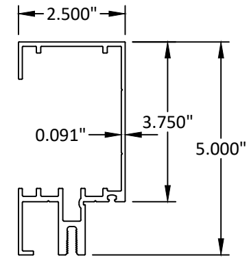
19 JAMB FOR 1" GL 6063-T5
