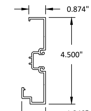
50 DOOR JAMB 6063-T5
