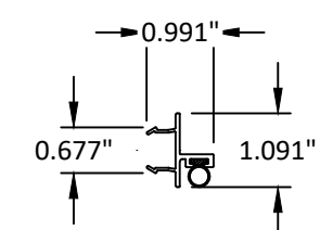
52 DOOR STOP 6063-T5
