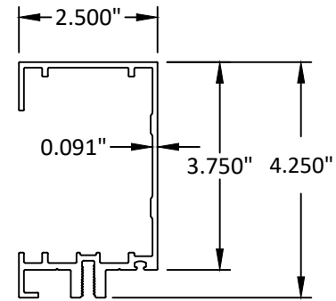
7 JAMB FOR 1/4" GL 6063-T5
