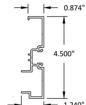
51 DOOR JAMB 6063-T5
