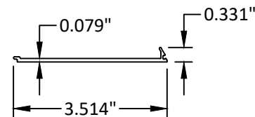
25 HORIZONTAL FLUSH FILLER 6063-T5
